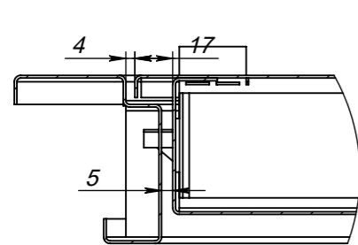
МЕСТНЫЙ L МАСШТАБ 1:3
